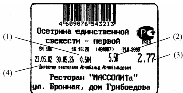
Рис. 12. Пример печати этикетки формата 45. Этикетка размером 58 x 40 мм. Когда препринта нет, числовые значения веса (1), цены (2) и стоимости (3) остаются "безымянными". (4) – сообщение, одна первая строка.
