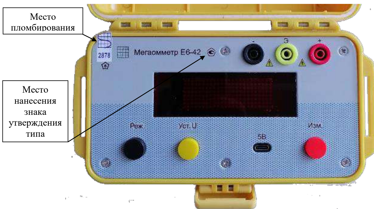
Рисунок 3 – Общий вид мегаомметров Е6-42
