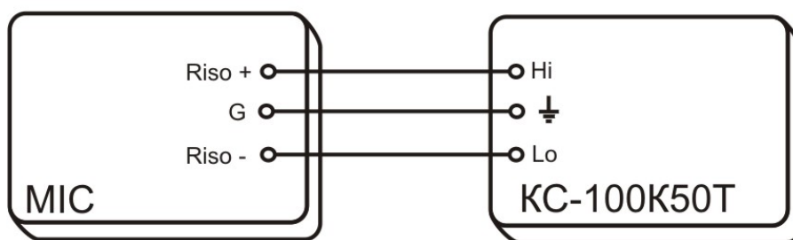
Рисунок 2 – Структурная схема определения абсолютной погрешности измерения сопротивления электроизоляции, где МІС – поверяемый измеритель, КС-100К5Т – калибратор электрического сопротивления.
