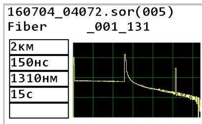
Рис. 20 Сохранённая рефлектограмма
