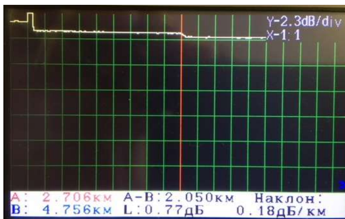
Рис. 18. Просмотр события 2 на графике рефлектограммы
