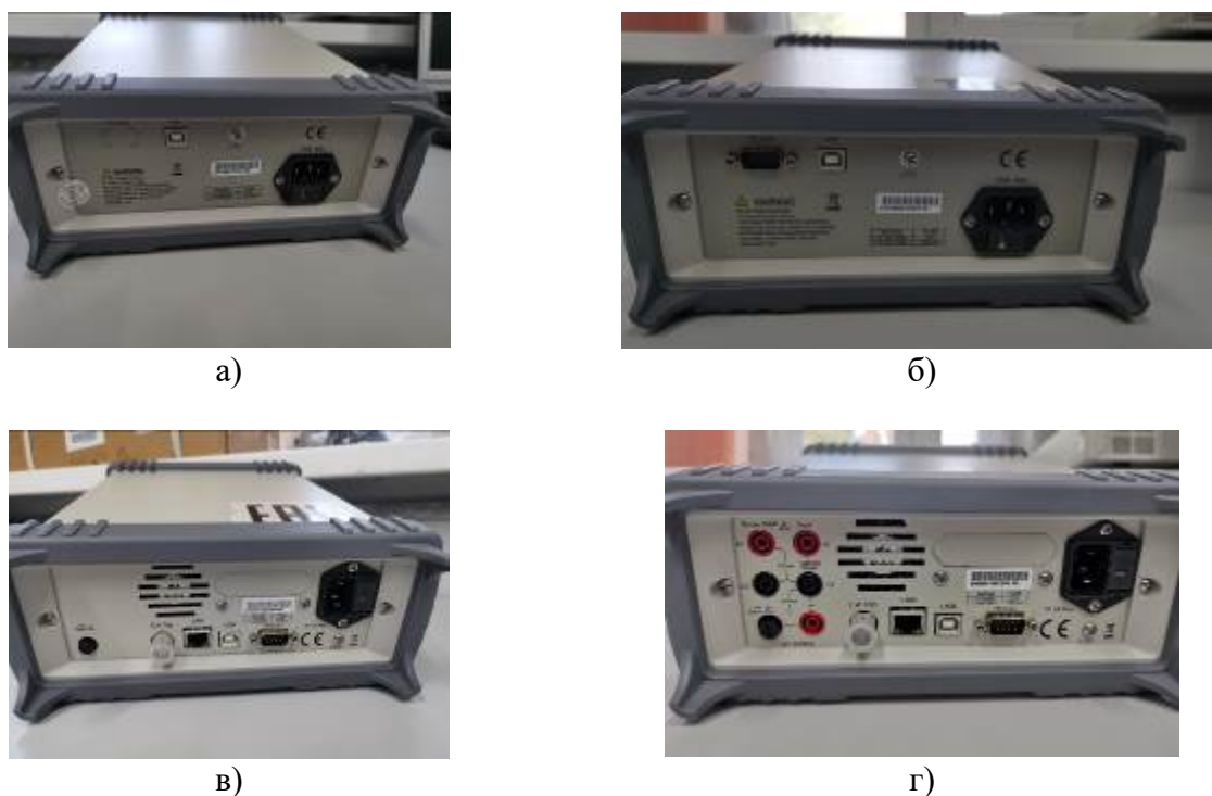
Рисунок 2 – Внешний вид (задняя панель) мультиметров VERDO MB2100 а) MB2101; б) MB2102; в) MB2105, MB2107; г) MB2106
