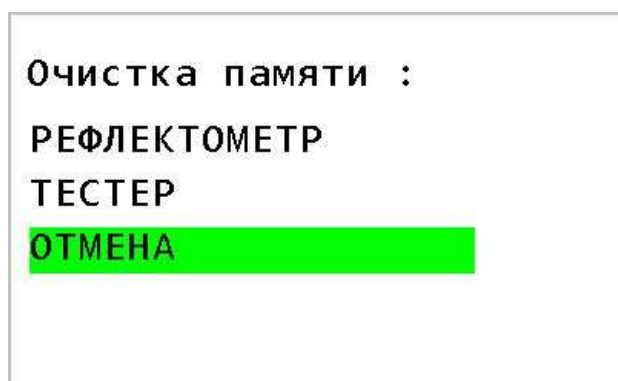
Рис. 33 Очистка памяти.
