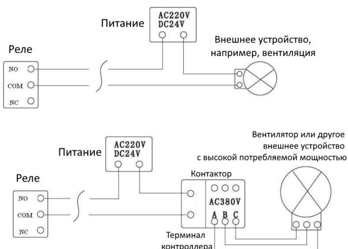
Подключение детектора и внешнего устройства
