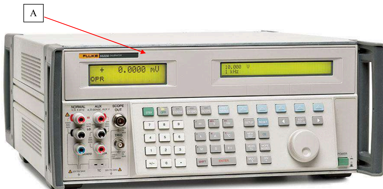
Рисунок 1 – Внешний вид калибраторов, место нанесения знака утверждения типа (А)
