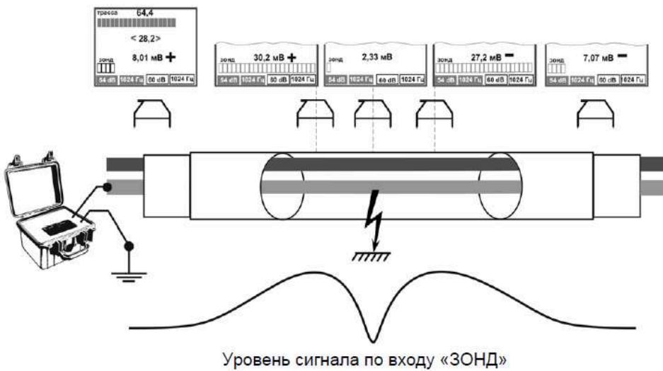
Рисунок 5.3.2 – Схема подключения и уровень сигнала при поиске замыкания жилы на броню
