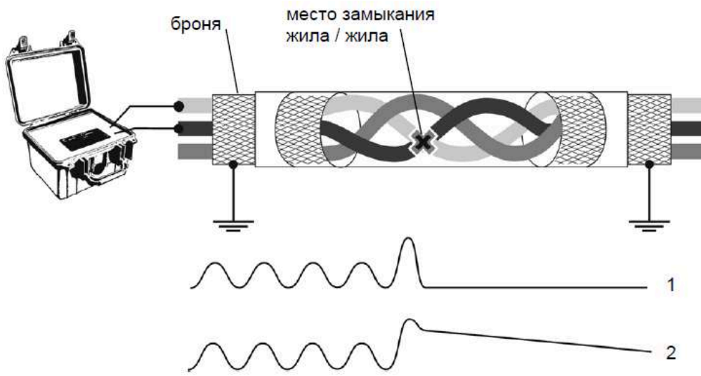
Рисунок 5.3.1 – Схема подключения и уровень сигнала при поиске замыкания между жилами
