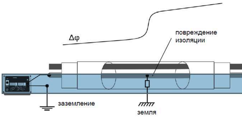
Рисунок 5.3.3.2 – Схема подключения и сдвиг фазы при поиске повреждения изоляции фазовым методом
