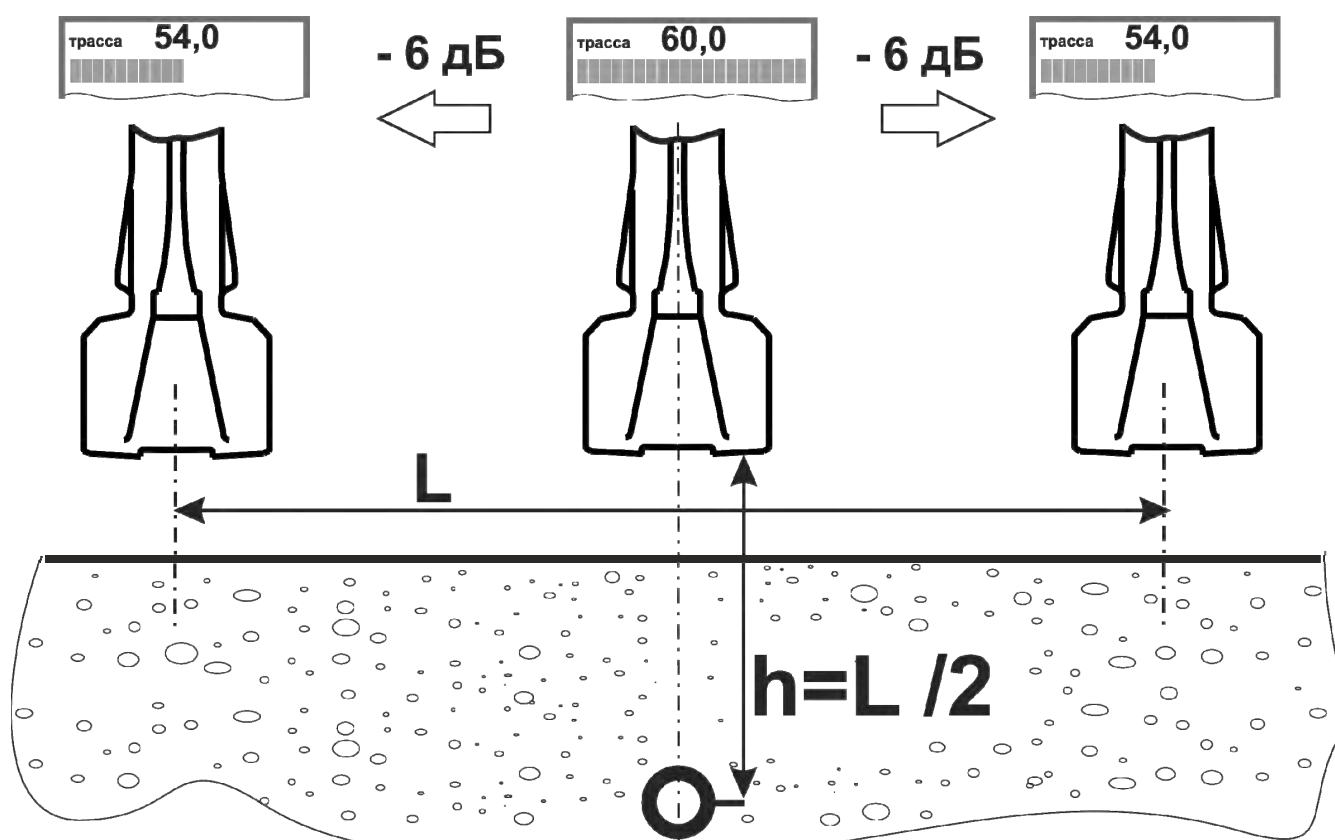
Рисунок 4.3.1 – Определение глубины залегания методом «-6дБ»
