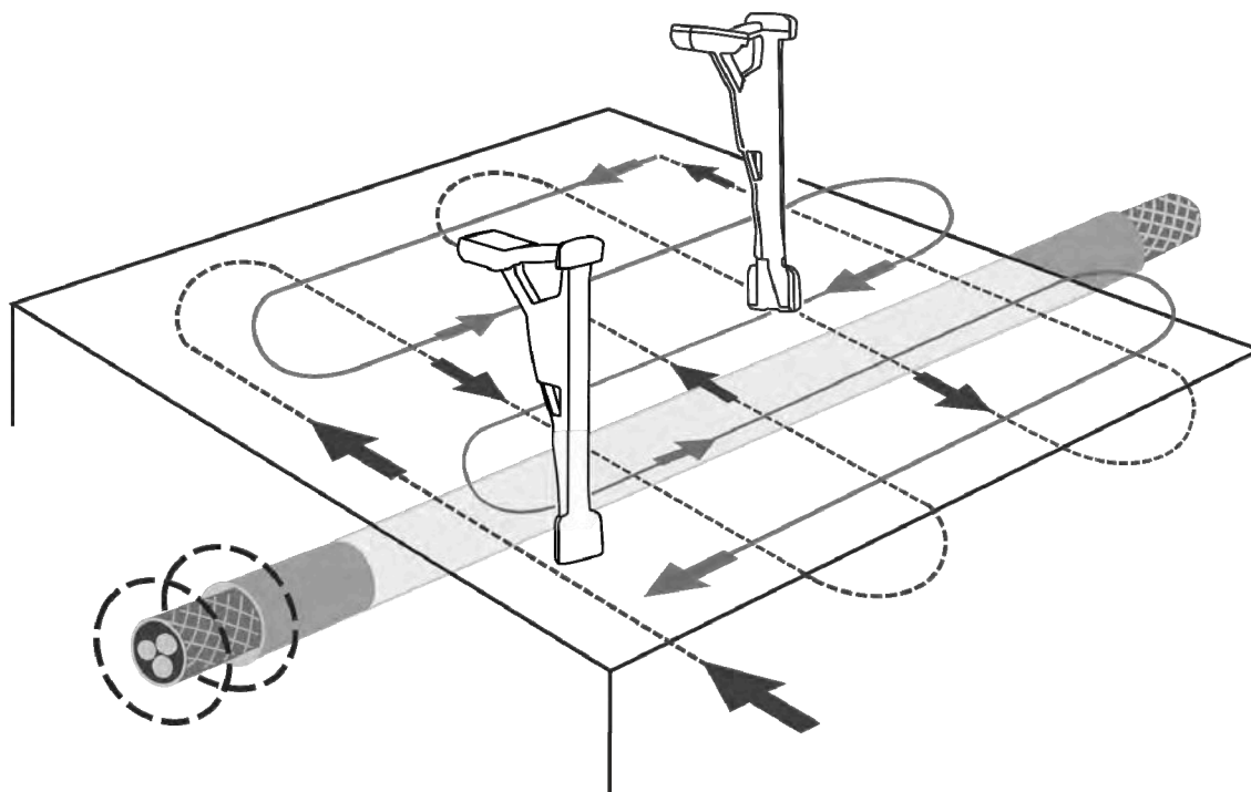
Рисунок 4.4.1 – Обследование участков местности без генератора
