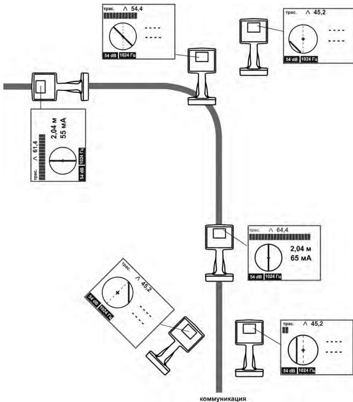
Рисунок 4.2.3а – Поиск с включенной функцией «КОМПАС»
