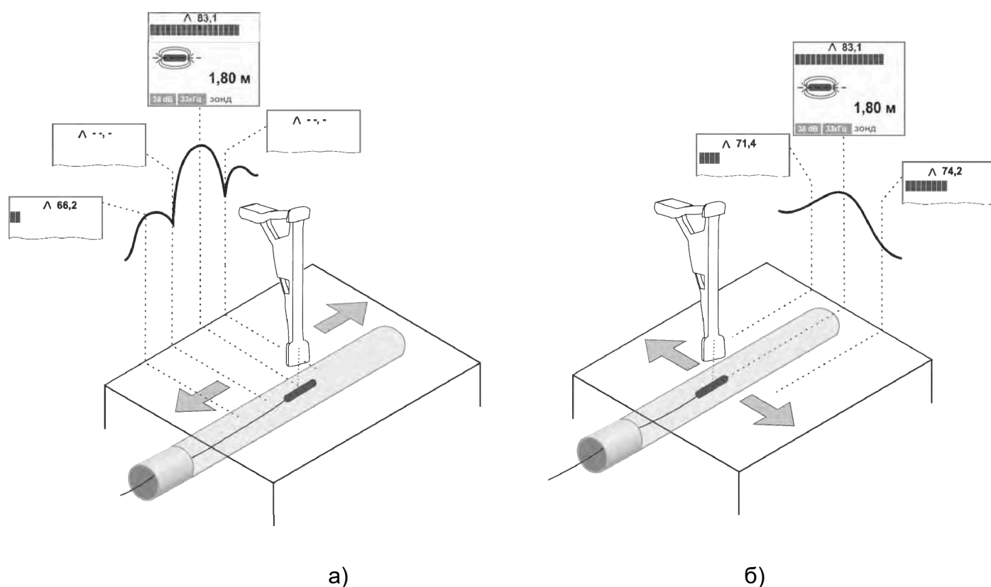
Рисунок 4.5.2 – Определение точного положения и глубины залегания зонда
