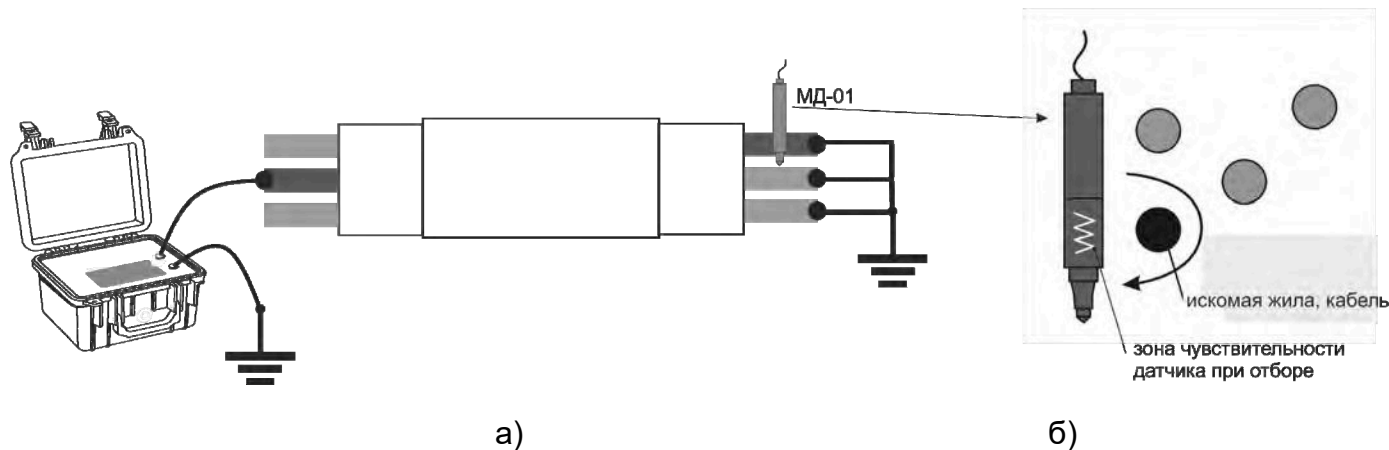
Рисунок 5.4.1 – Схема подключения при отборе жил кабеля
