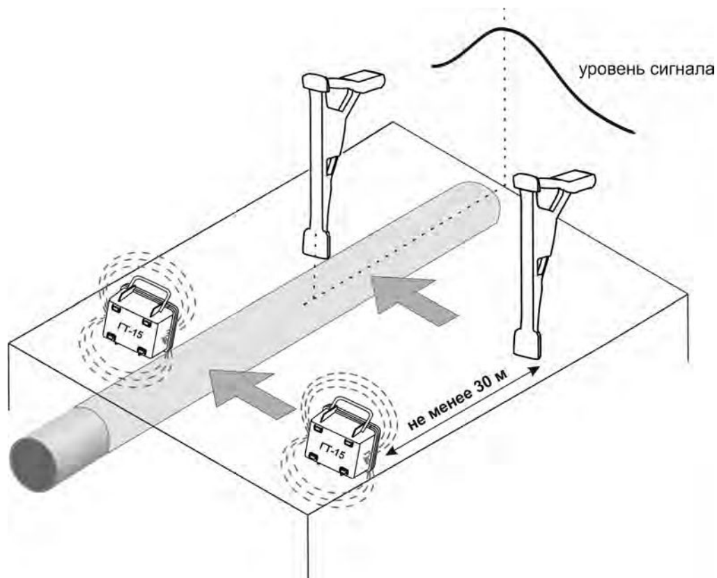
Рисунок 4.4.2 б – Обследование участков местности с помощью ГТ-15
