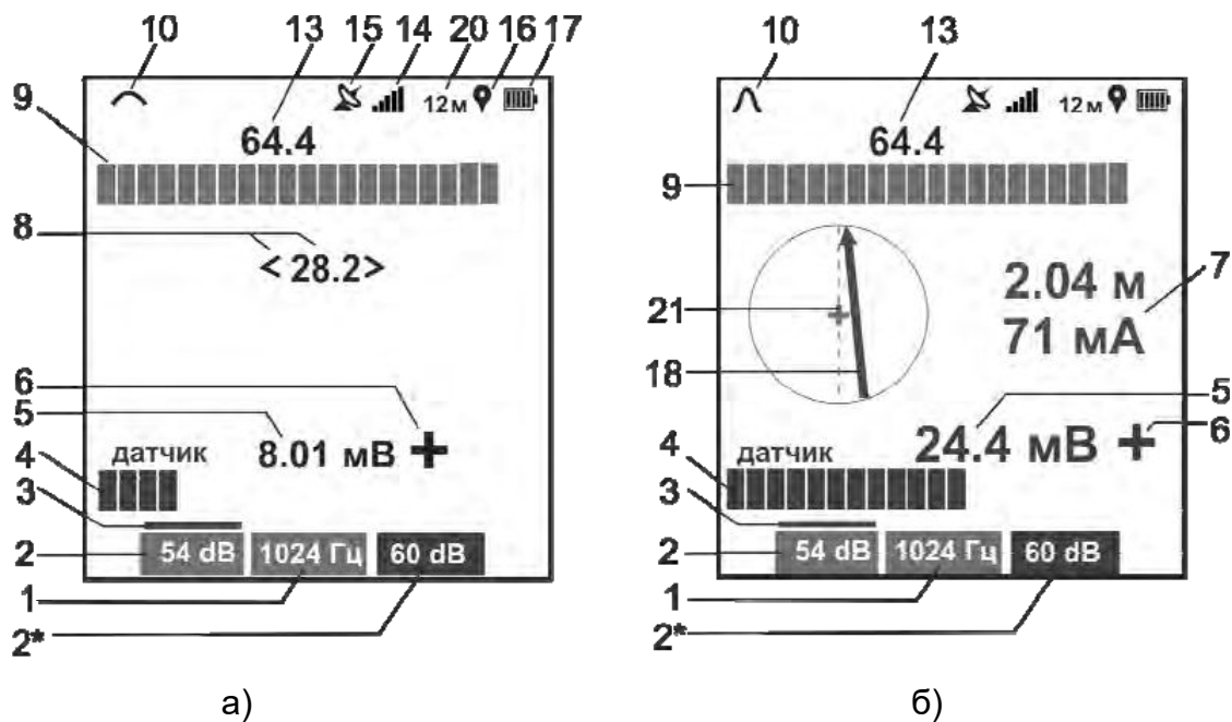
Рисунок 3.3 – Индикация приемника в режиме «ТРАССА-ДАТЧИК»
