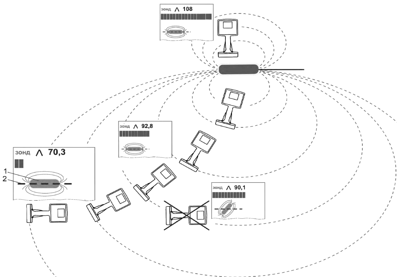
Рисунок 4.5.1 – Поиск местоположения зонда
