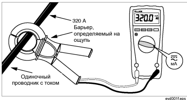
Рис. 1. Измерение тока
