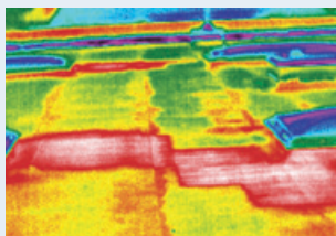
Изображение, выдаваемое тепловизионной камерой
