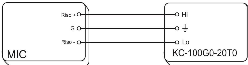
Рисунок 3 - Структурная схема определения абсолютной погрешности измерения сопротивления электроизоляции при номиналах сопротивлений до 20 ТОМ с испытательным напряжением до 10 кВ.
